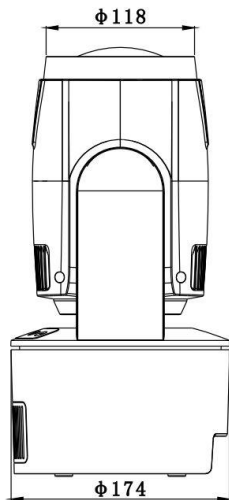
侧面图
