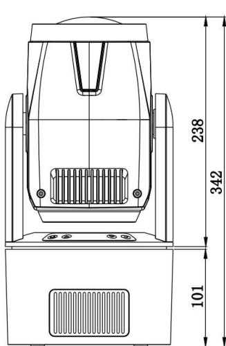
正面图
