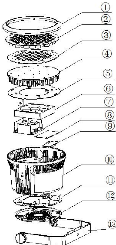
附 1：灯具结构分解图
