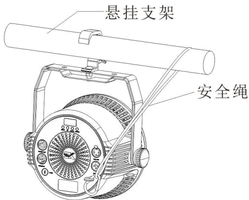
图（4.2-2）：安全绳安装图
