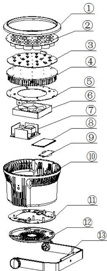
附 1：灯具结构分解图
