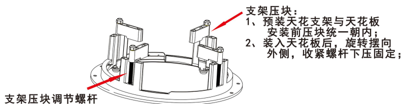
预装天花支架
