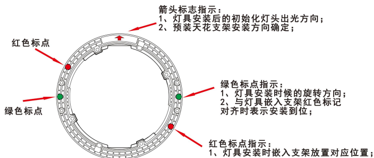
预装天花支架
