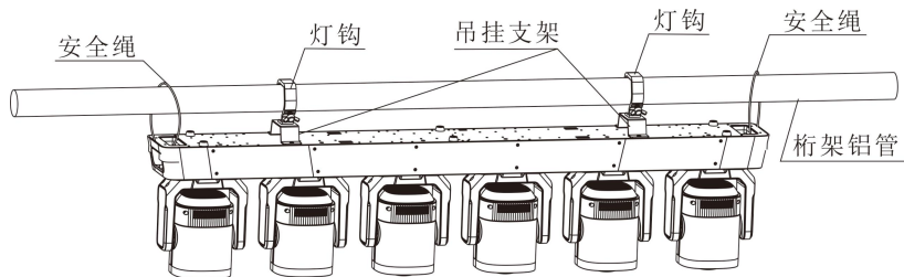
灯钩吊挂安装效果图
