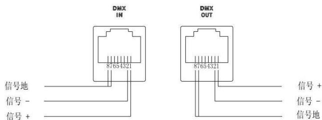
RJ45座接口、电源接口
