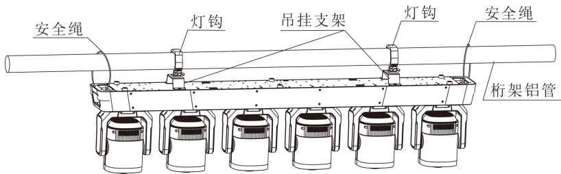
灯钩吊挂安装效果图
